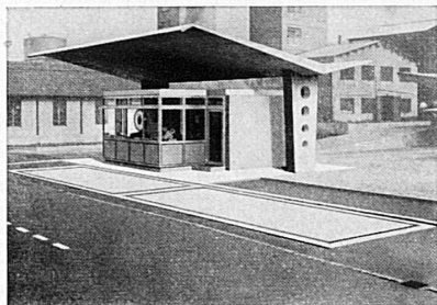
Automatische Verbund-Brückenwaage für Straßenfahrzeuge. Wägefähigkeit 30 t. Es kann mit jeder Brücke einzeln oder mit beiden zusammen gewogen werden.
