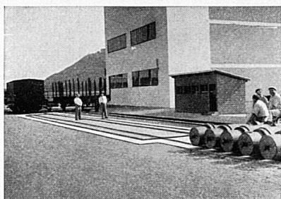
Brückenwaage für Geleisefahrzeuge. Wägefähigkeit 200 000 kg, Brückenlänge 24 m, Brücke in vorgespanntem Beton mit nur 4 Auflagern. Anlässlich der amtlichen Eichung ergab sich ein maximaler Fehler in der Gewichtsanzeige von nur 1-9 kg. Die Empfindlichkeit bei Vollast betrug 2 kg.
