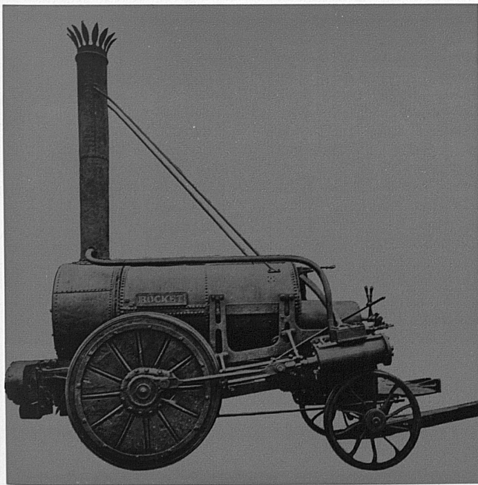
Die «Rocket» im schlechten Zustand von 1862, als sie das Britische Patentamt erhielt: Sie war für den Dienst in einer Mine verstärkt worden.
