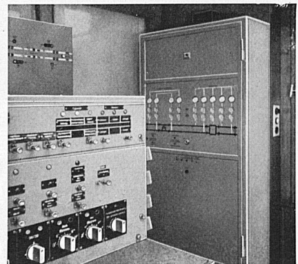
Fernsteuerungsanlage, Bahnhof Göschenen
