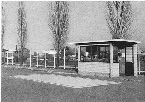
Abbildung: Fuhrwerkswaage 40 000 kg Brückengröße 10 x 3,2 m Laufgewichtsbalken mit Messkopf kombiniert
