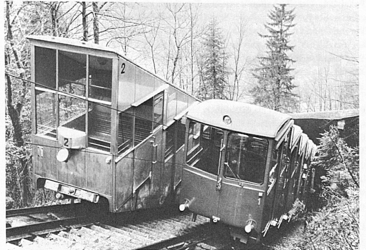
Neue und alte Standseilbahnkabine der Stoosbahn. Abschluss der Totalerneuerung Sommer 1970.
