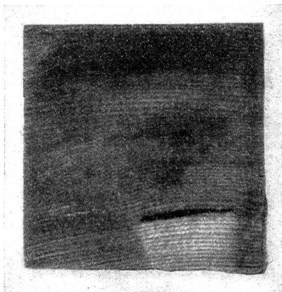
Phot. A. Bourquin, Zürich. N° 4. Base d'un parallépipède employé pour un essai de résistance à la pression dans le sens des fibres (grand. nat.).
