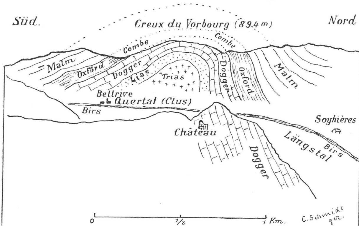
Fig. 4. Gewölbe der Vorbourg-Kette bei Soyhières.
