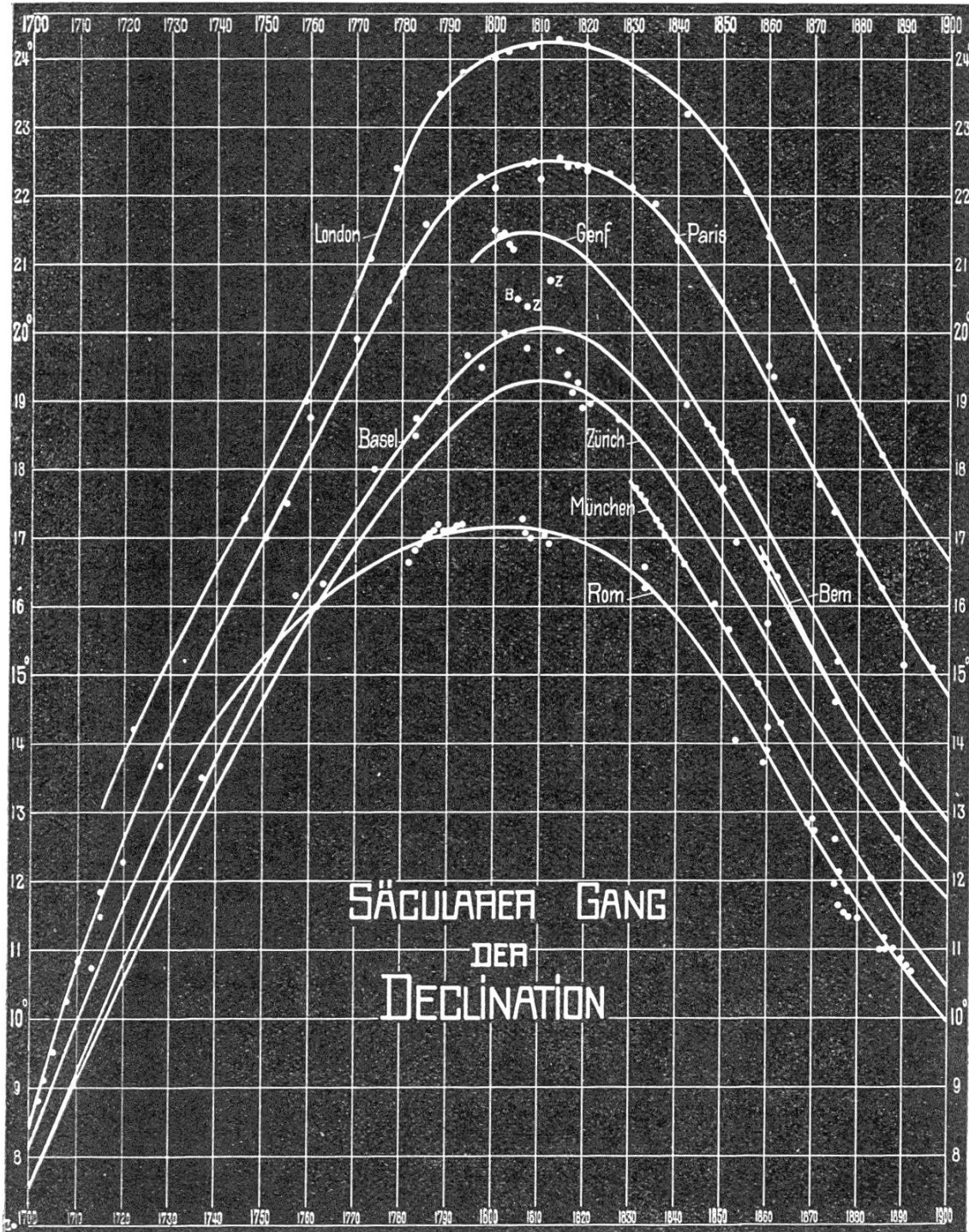
Die Änderung (Säkularvariation) der magnetischen Declination in der Schweiz und Umgebung von 1700—1900.
