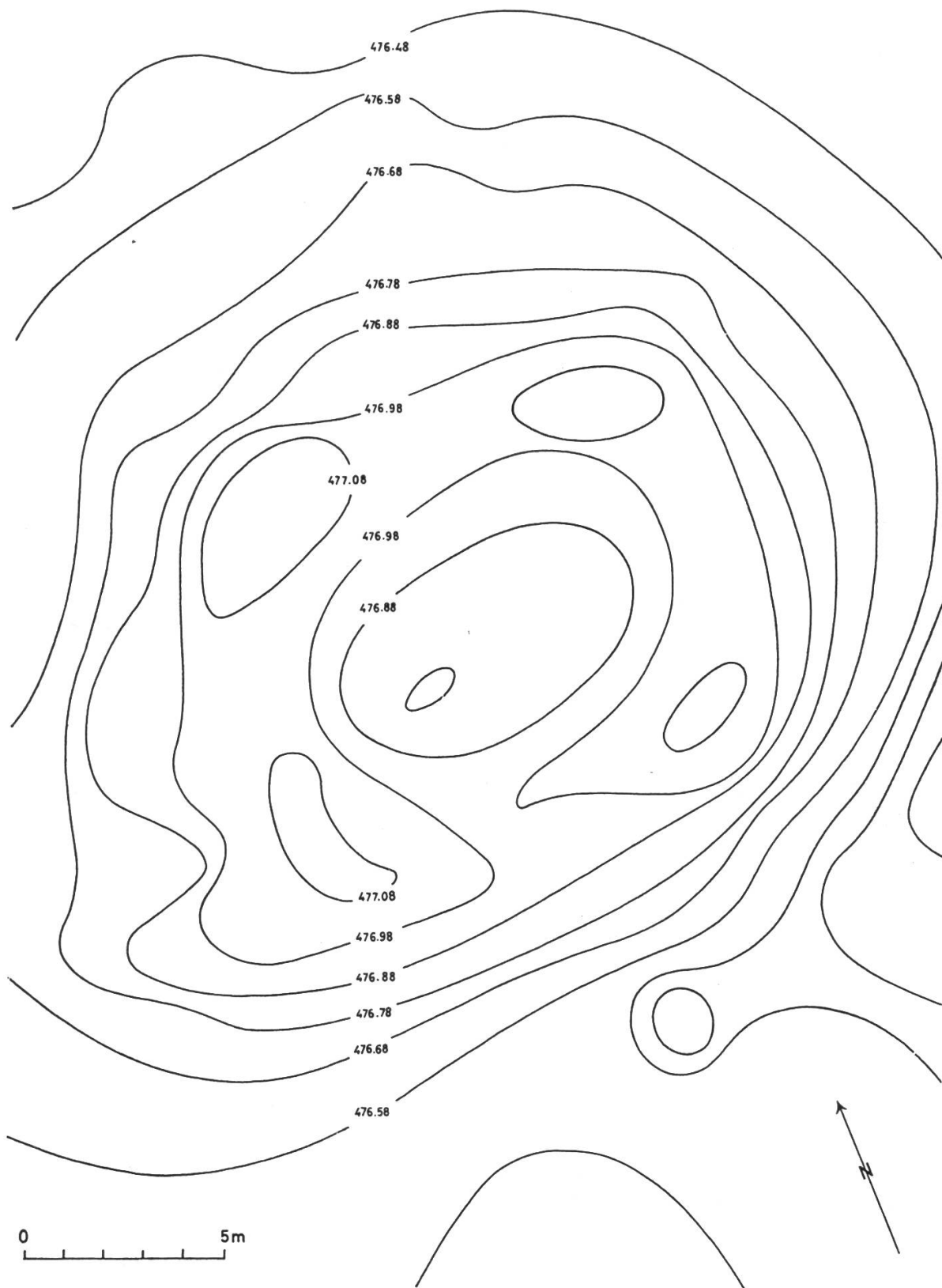
Abbildung 5. Riehen-Maienhühl: 10-cm-Höhenkurvenplan von Punkt 477 (618 200/271 550). Die Ecken des Gebäudes sowie die Türöffnung auf der Südseite lassen sich schon deutlich ablesen. Vergleiche Abbildung 6. — Massstab 1 : 200.
