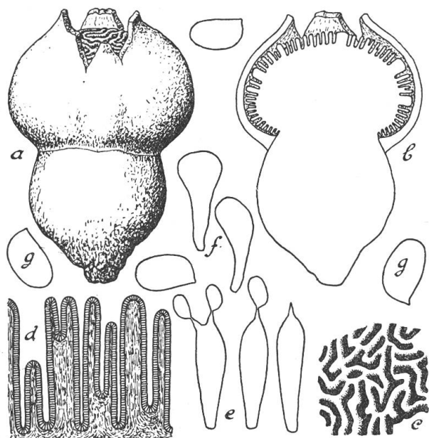
Fig. 2. — Anomalie d' Agaricus campester Fr., forme cultivée. — a, carphore; gr. nat. — b, coupe; gr. nat. — c, aspect de l'hyménium vu par-dessus; \times 3,5 . — d, coupe verticale de l'hyménium; \times 6 . — e, basides; \times 500 . — f, cellules différenciées de l'arête des lames; \times 500 . — g, spores; \times 1000 .
