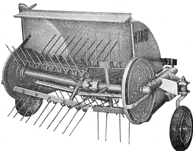
Epandeuse d'herbe Wängi
