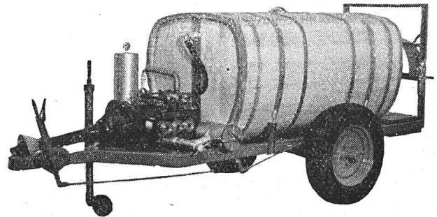
Pulvérisateur à haute pression Royal, pour prise de force
