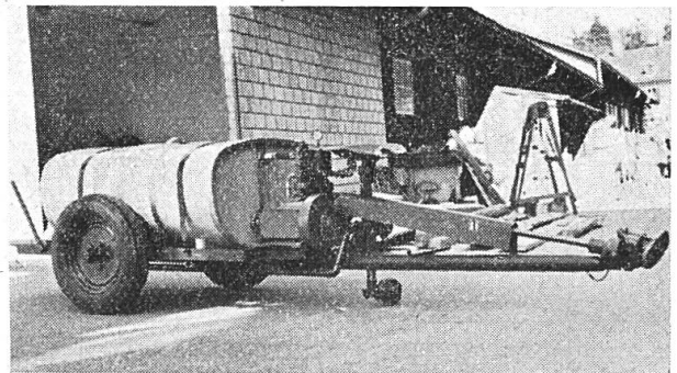
Autre pulvérisateur à haute pression Royal, pour prise de force.
