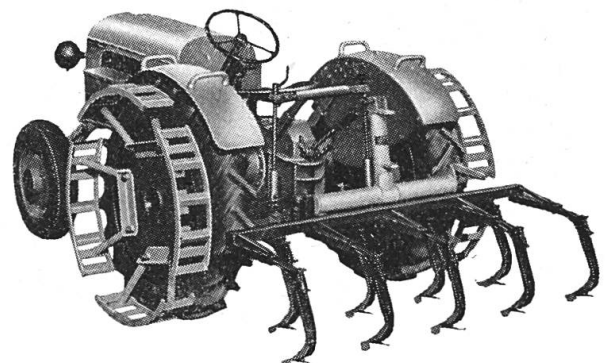
Roues d'adhérence Meili et cultivateur
