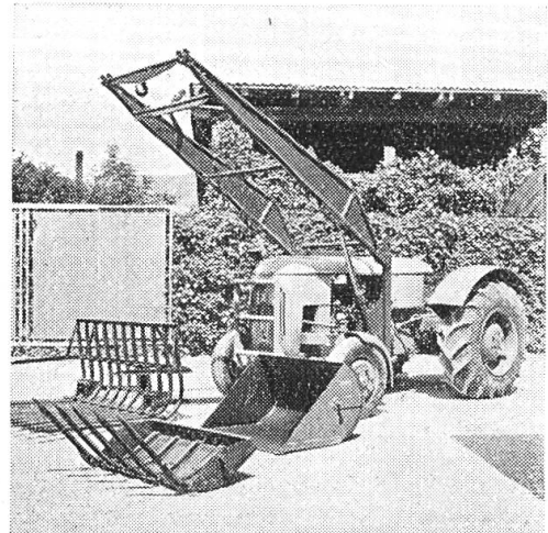
Chargeur frontal Wittenburg-Vevey
