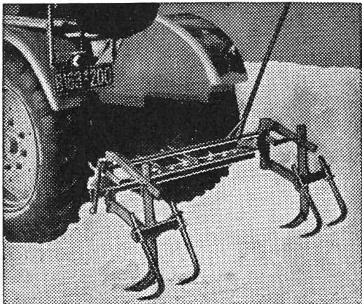
Griffes fousseuses Degenhart (Griesser, Andelfingen/ZH)
