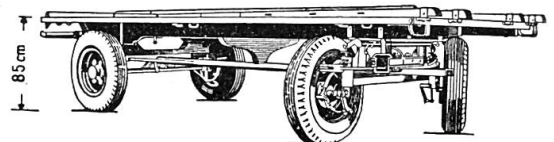
Remorque à deux essieux Neuhaus
