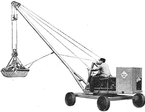
Grue à fumier Mengele
