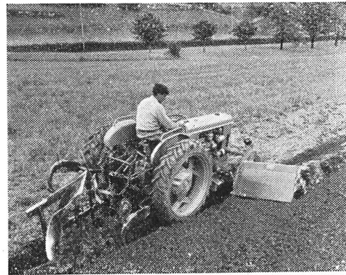
Herse rotative portée Vevey à montage latéral
