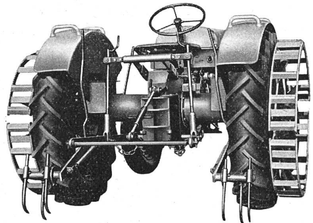
Roues d'adhérence et griffes fousseuses Meili
