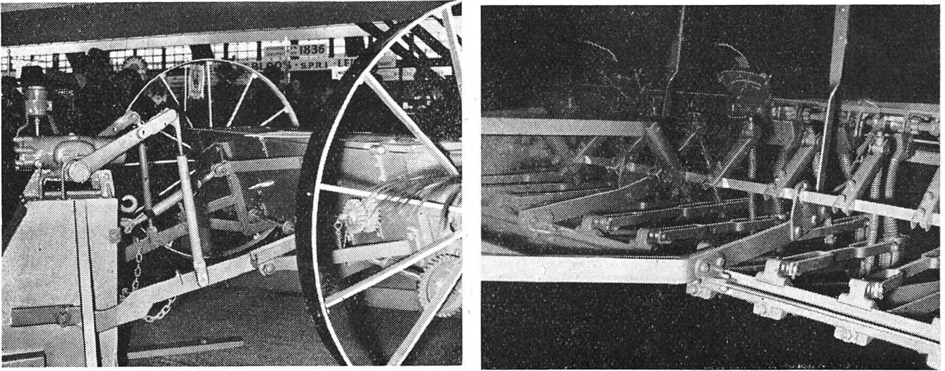
Fig. 1: Le nouveau relevage hydraulique «Fendt», pour attelage en 3 points. Derrière: épandeur d'engrais à plateaux «Melotte». X. Fendt, Marktobersdorf/Allgäu (All.). Melotte SA, Gembloux (Belgique).
