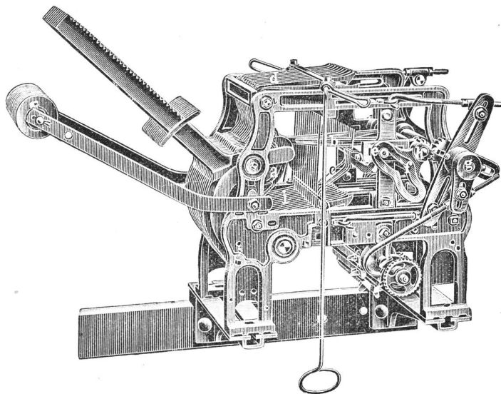
2 cylindrige Schaftmaschine
