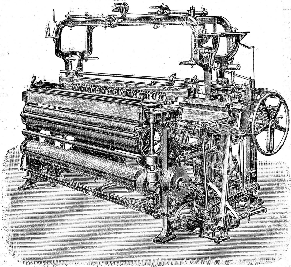
Einschützigter Brochierwebstuhl mit Kreislade.
