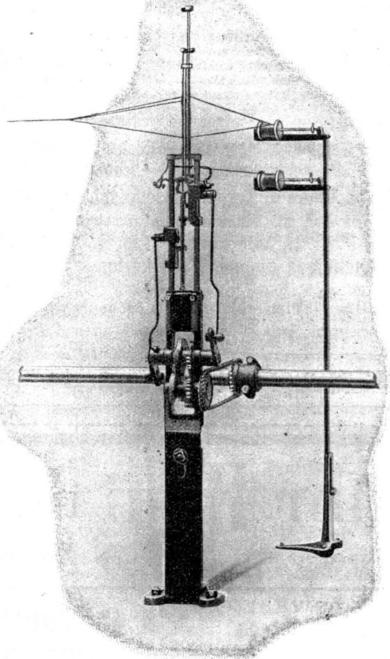
Antrie von der Excenterwelle.
