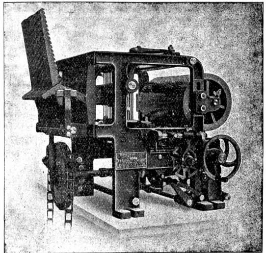
Doppelhub-Schafmaschine „Reform“
