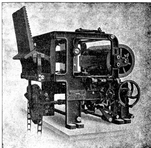
Doppelhub-Schafmaschine „Reform“
