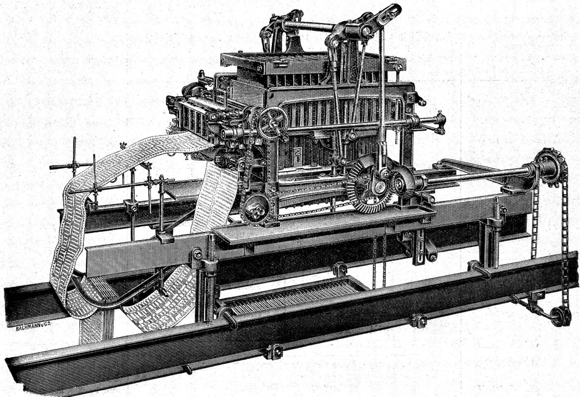
Doppelhub-Verdolmaschine für hohe Arbeitgeschwindigkeit besonders geeignet
