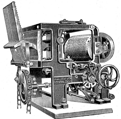
Doppelhub-Schaftmaschine „Reform“
