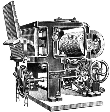
Doppelhub-Schafftmaschine „Reform“
