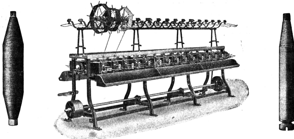
Kreuzschußpulmaschine „RAPID“, die bestkonstruierte und leistungsfähigste Schuß-Spülmaschine der Gegenwart
