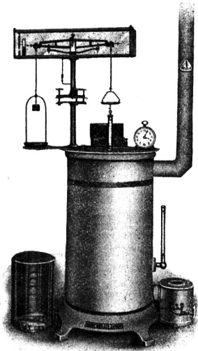
Gangbarste Größe: Für Versuche bis 500 gr. und mehr. Zur Bestimmung des Feuchtigkeitsgehaltes loser Textil-Rohstoffe und Garne von Wolle, Seide, Baumwolle, (Papier-Rohstoffe, Holzschliff etc.). Für Spiritus-, Gas- oder elektrische Heizung. Neueste solide Ausführung mit feinsten Präzisions- Wage in metallgefasstem Glasgehäuse, Drahtkorb, Hakenkranz, Thermometer, Wasserwage, Gewichtssatz
