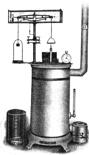
Gängbarste Grösse: Für Versuche bis 500 gr. und mehr. Zur Bestimmung des Feuchtigkeitsgehaltes loser Textil-Rohstoffe und Garne von Wolle, Seide, Baumwolle, (Papier-Rohstoffe, Holzschiiff etc.). Für Spiritus-, Gas- oder elektrische Heizung. Neueste solide Ausführung mit feinsten Präzisions- Wage in metallgefasstem Glasgehäuse, Drahtkorb, Hakenkranz, Thermometer, Wasserwage, Gewichtssatz
