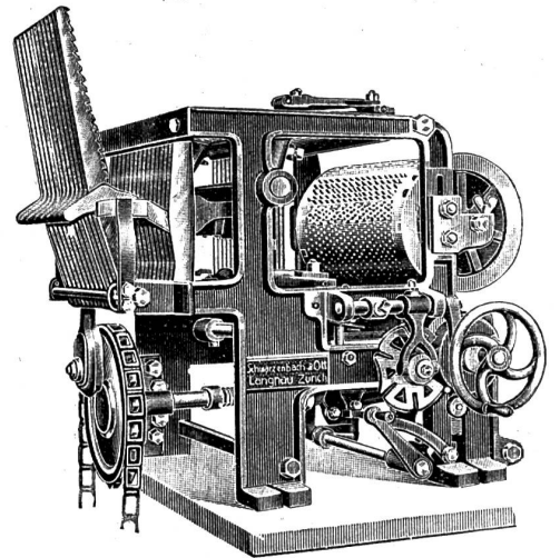
Doppelhub-Schaffmaschine „Reform“
