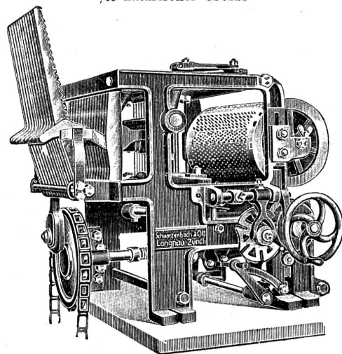
Doppelhub-Schafmaschine „Reform“
