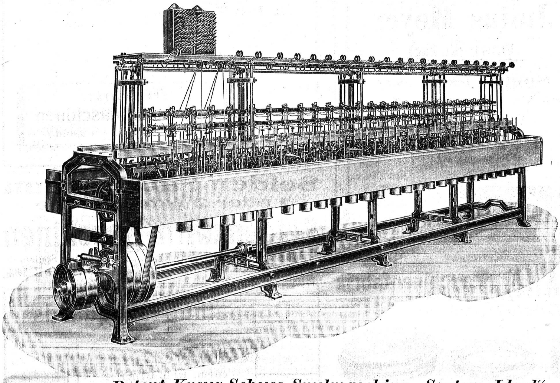
Patent-Kreuz-Schuss-Spülmaschine „System Ideal“
