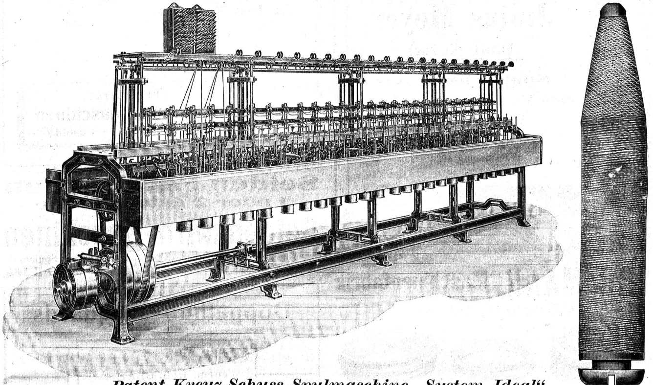
Patent-Kreuz-Schuss-Spülmaschine „System Ideal“
