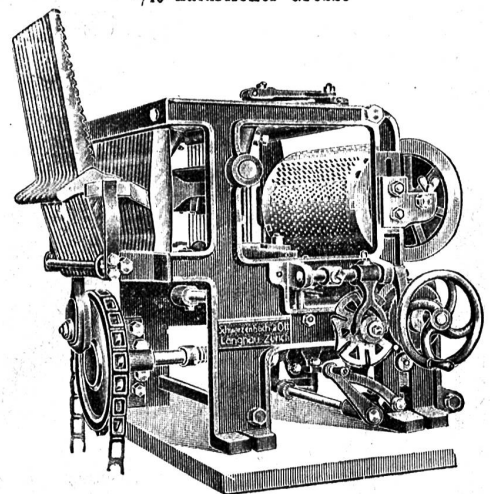
Doppelhub-Schaftmaschine „Reform“
