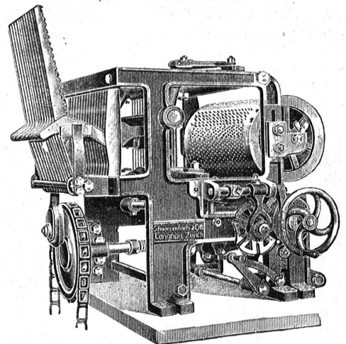
Doppelhub-Schaftmaschine „Reform“
