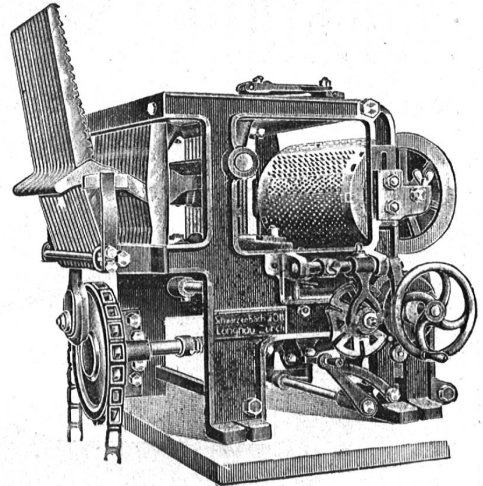
Doppelhub-Schafmaschine „Reform“
