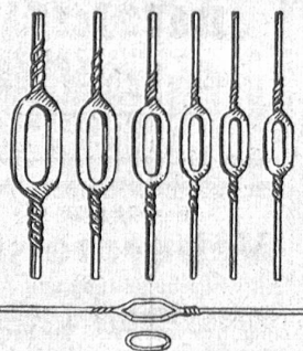
Universallitzen mit eingesetztem Stahling
