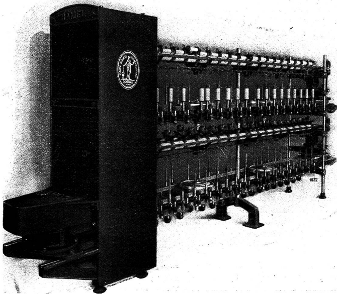
Etagenzwirmaschine Modell LL 65.
