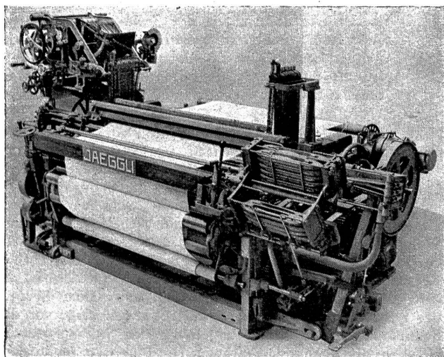
Seidenwebautomat
