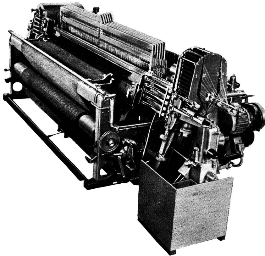
Abb. 1 Universal-Lancier-Automatenwebstuhl Typ «JURA» Automatische Seite
