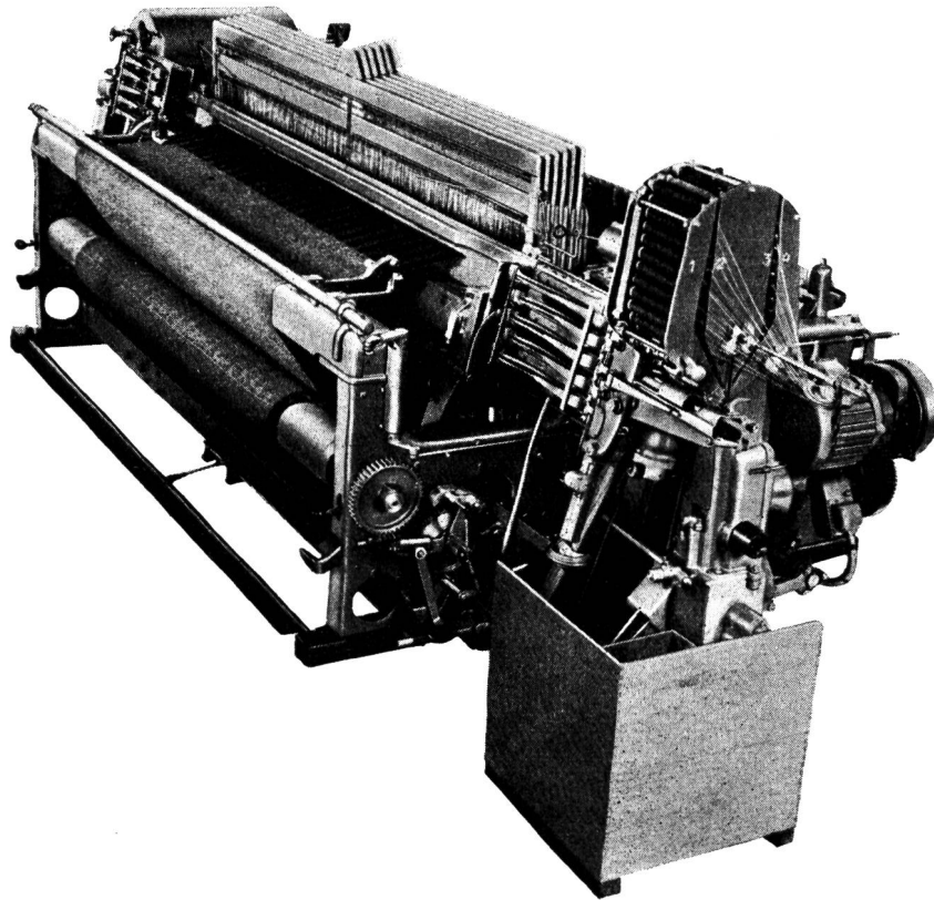
Abb. 1 Universal-Lancier-Automatenwebstuhl Typ «JURA» Automatsseite
