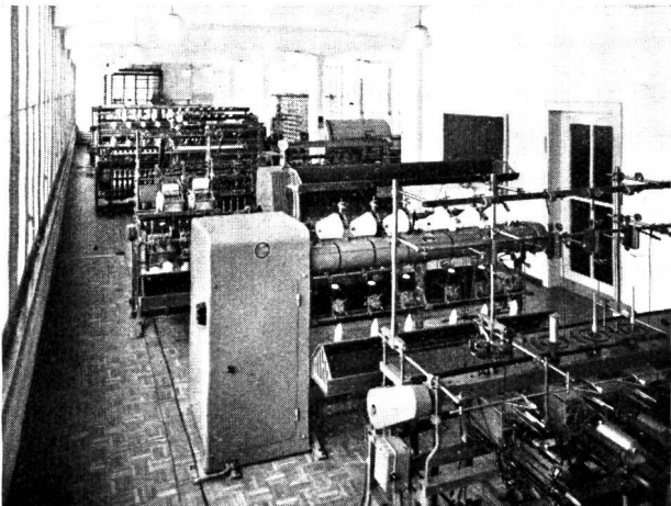
Weberei-Vorwerkmaschinen
