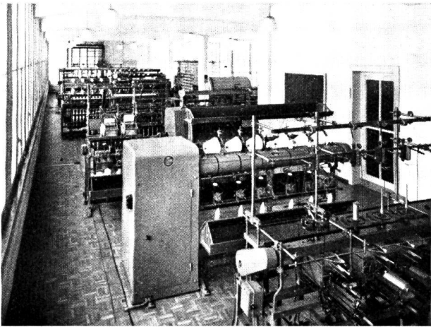
Weberei-Vorwerkmaschinen
