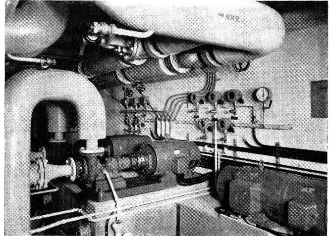
Schindler-Ward-Leonhard-Umformergruppe und Gleichstrom-Nebenschluß-Motoren röhrengesteuerter Pumpenantriebe mit automatischer Regelung auf konstanten Druck
