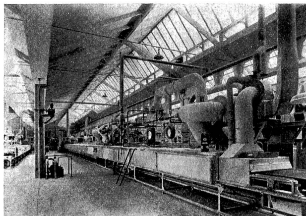
Vulkanisierungsapparat
