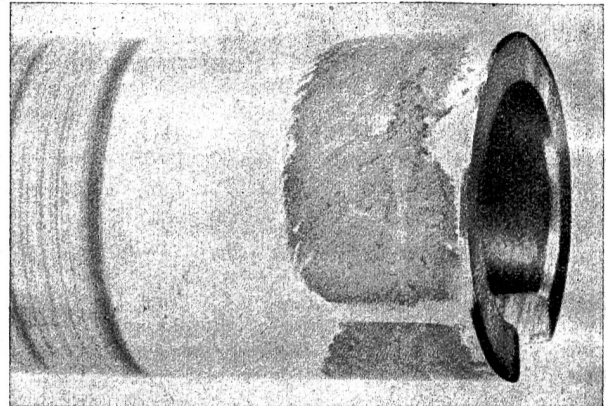
Abb. 4: Besonders gut «gewachsener» Passungsrost an der Einspannstelle eines zylindrischen Prüfkörpers hoher Oberflächengüte ( \mu max. = 0,2 ). Der schmale, rechts sichtbare Steg ohne Passungsrost ist durch die Spannzange entstanden (Schlitz in der Spannzange). Farbe der Aufwachsung braunrot, also ist der Passungsrost älteren Datums (Sekundärform).
