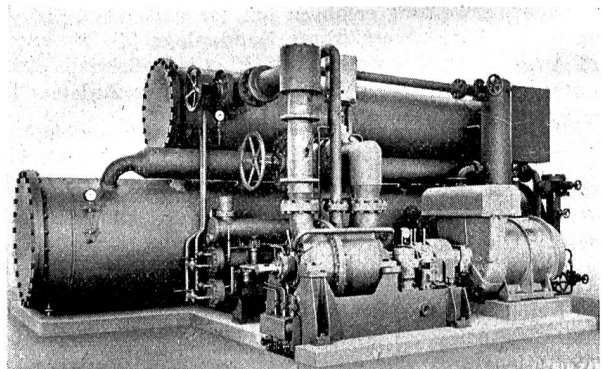
Charakteristisch für die Uniturbo-Kältemaschine sind die raumsparende Blockeinheit und die kompakte, doch übersichtliche und leicht zugängliche Anordnung von Turbo-kompressor, Elektromotor, Kondensator und Verdampfer.
