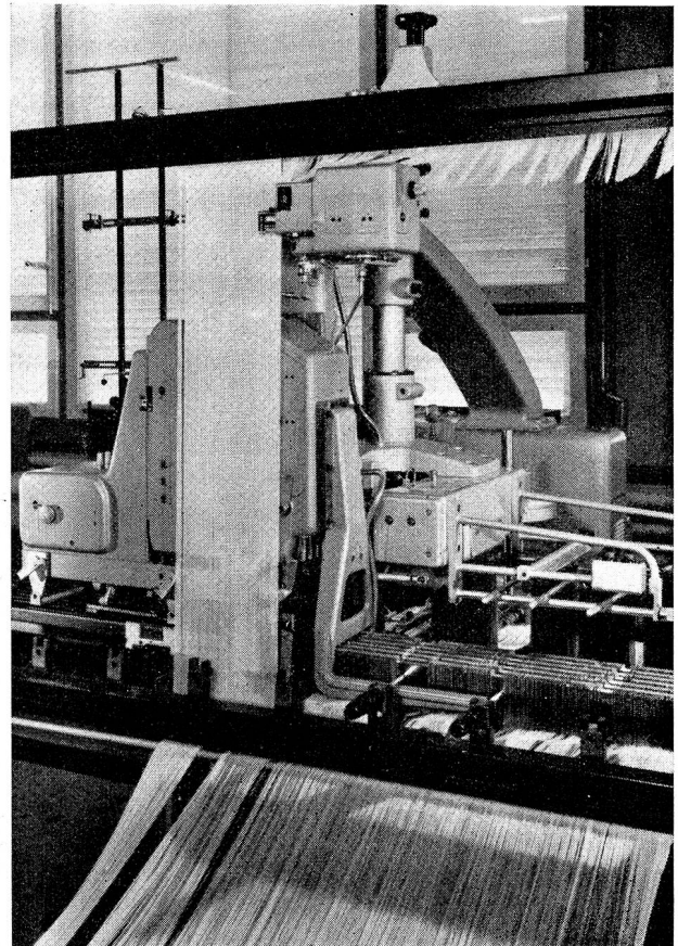
Automatische Einziehmaschine USTER Typ EMU 31
