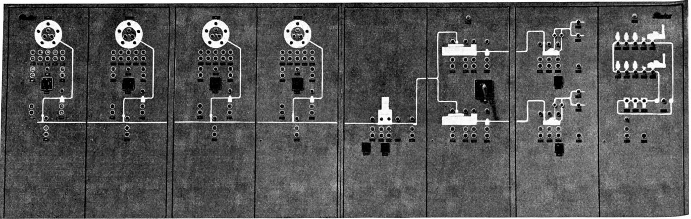
Schaltzentrale für die elektropneumatische Steuerung der Oeffnungs- und Reinigungsmaschinen (Bild 8)
