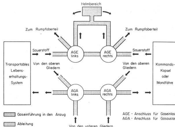
Abb. 3 Druck- und Ventilationssystem in schematischer Darstellung
