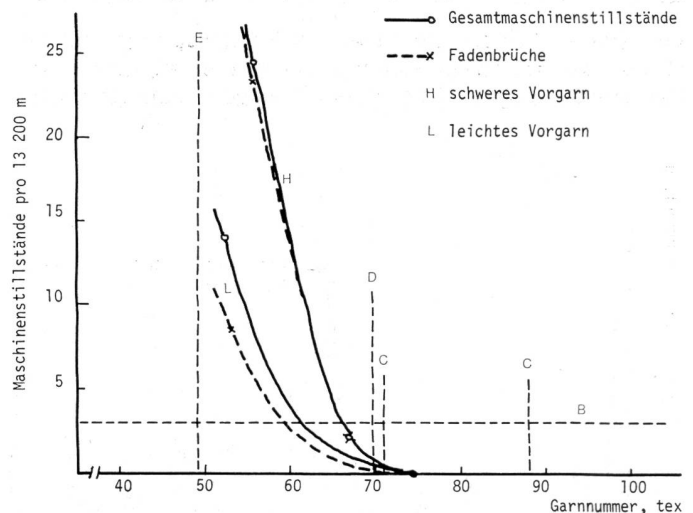
Abbildung 4 Spinnverhalten von 25,8 \mu -Vorgarnen
