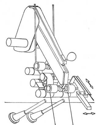
Abbildung 17 Einlegen des Fadenendes
