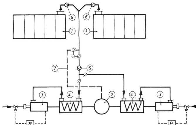
Thermische Abluftreinigung mit Abluftvorwärmung, Abluftregelbereich 1:4 – 1 Trockner, 2 Reinluftkamin, 3 Combustor, 4 Abluftvorwärmer, 5 Abluftventilator, 6 Abluftventilator, 7 Bypass-Leitung.
