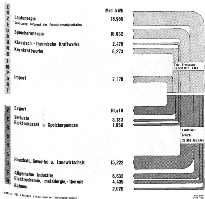
Abbildung 4 Erzeugung und Verbrauch an elektrischer Energie in der Schweiz (1972/73)
