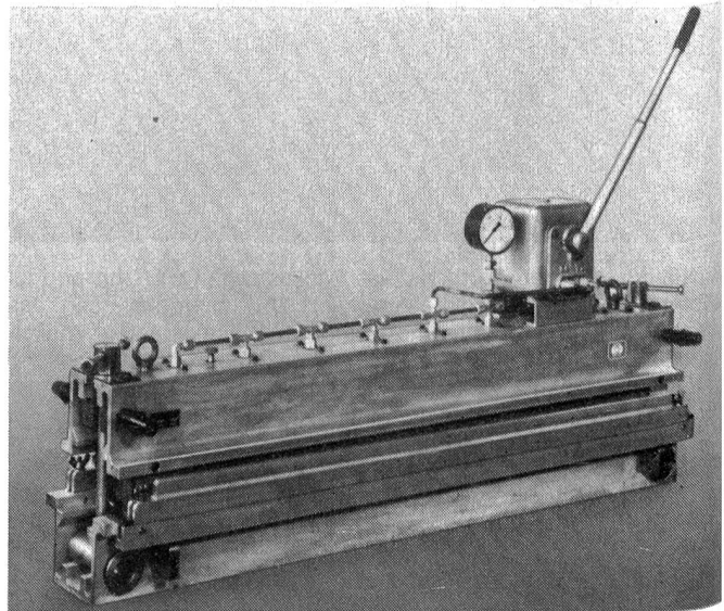
Abbildung 7 Hydraulisch spannbare Heizpresse zum Endverbinden der beiden Enden von Transportbändern. Von Bandfabrikanten gelieferte Spezialkleber ergeben unter Druck und Temperatur Endverbindungen, deren Qualität bezüglich Zugfestigkeit, Biegesteifigkeit etc. ausserordentlich gut ist (Typ aus dem Lieferprogramm der Habasit AG, verwendbar bis 1200 mm Bandbreite).
