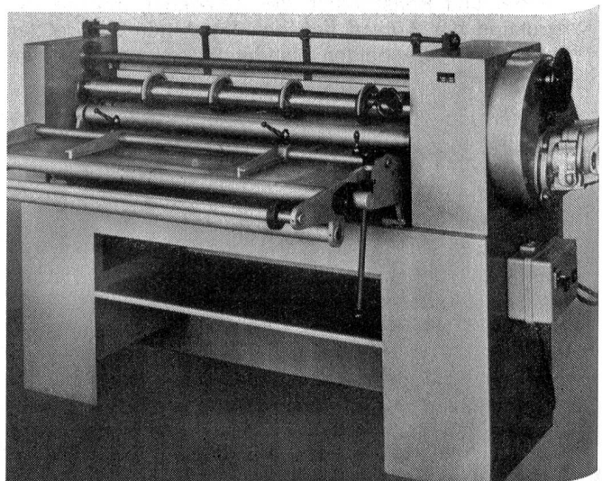
Abbildung 8 Maschine zum Schneiden von Transportbändern auf die benötigte Breite. Es können mehrere Schnitte gleichzeitig und in beliebigem Abstand ausgeführt werden. Die Maschine ist hier für vier Schnitte ausgerüstet (Messer auf der zweitobersten Walze). Der Vorschub des Bandes geschieht automatisch (Typ aus dem Lieferprogramm der Habasit AG, verwendbar bis 1200 mm Bandbreite).
