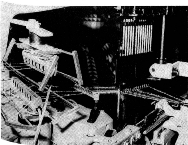
Steuerung zur Schussgarnvorlage an den Greifer
