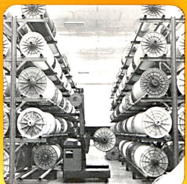
Universal-Seitenstapler
