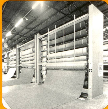
Teppichrollen-Paternoster
