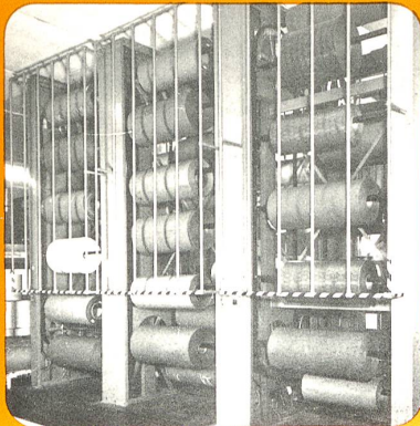
Folien-Paternoster
