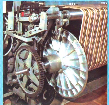
Dämmapparat mit Streichbaum
