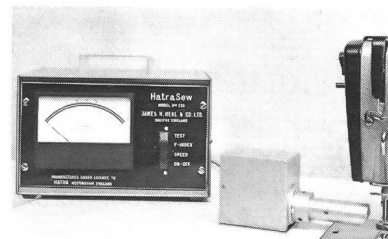
HATRASEW Stickschaden-Prüfgerät
